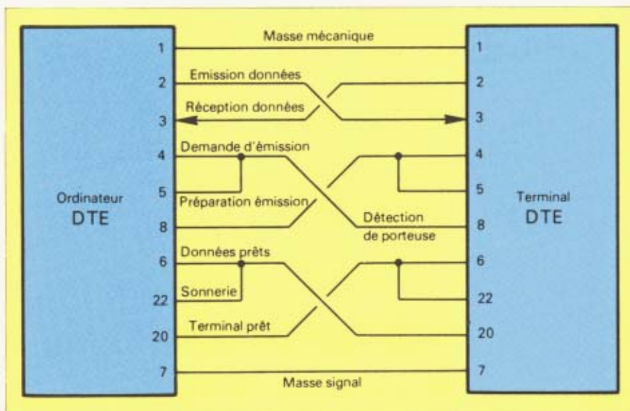
Le câble pour « modem nul » croise certaines connexions.
